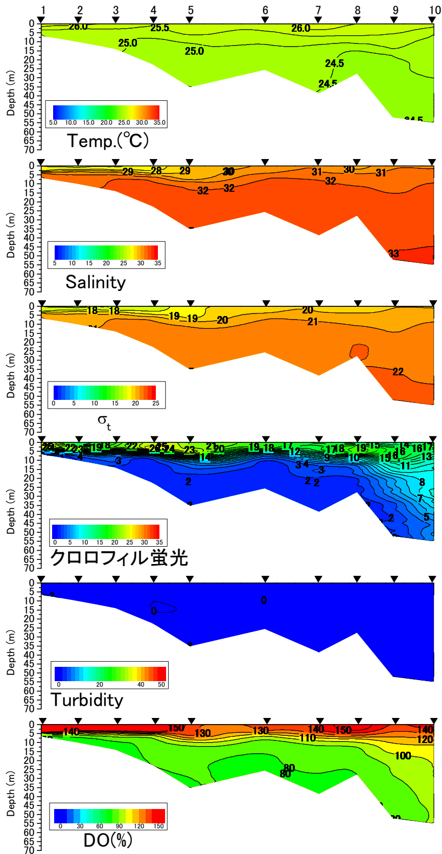
有明海中央ラインの水温(°C)、塩分、密度( \sigma_t )、クロロフィル蛍光強度、濁度、溶存酸素飽和度(DO%)の鉛直面図(国土交通省の調査による) (2016年9月27日)
